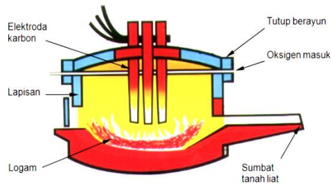
Gambar 1.5. Dapur Listrik Busur Cahaya
