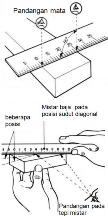
Gambar 3.2. Cara menggunakan mistar ukur
