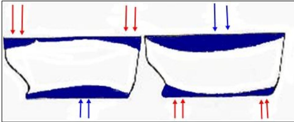
Gambar 23. Kondisi kapal akibat pemuatan membujur
