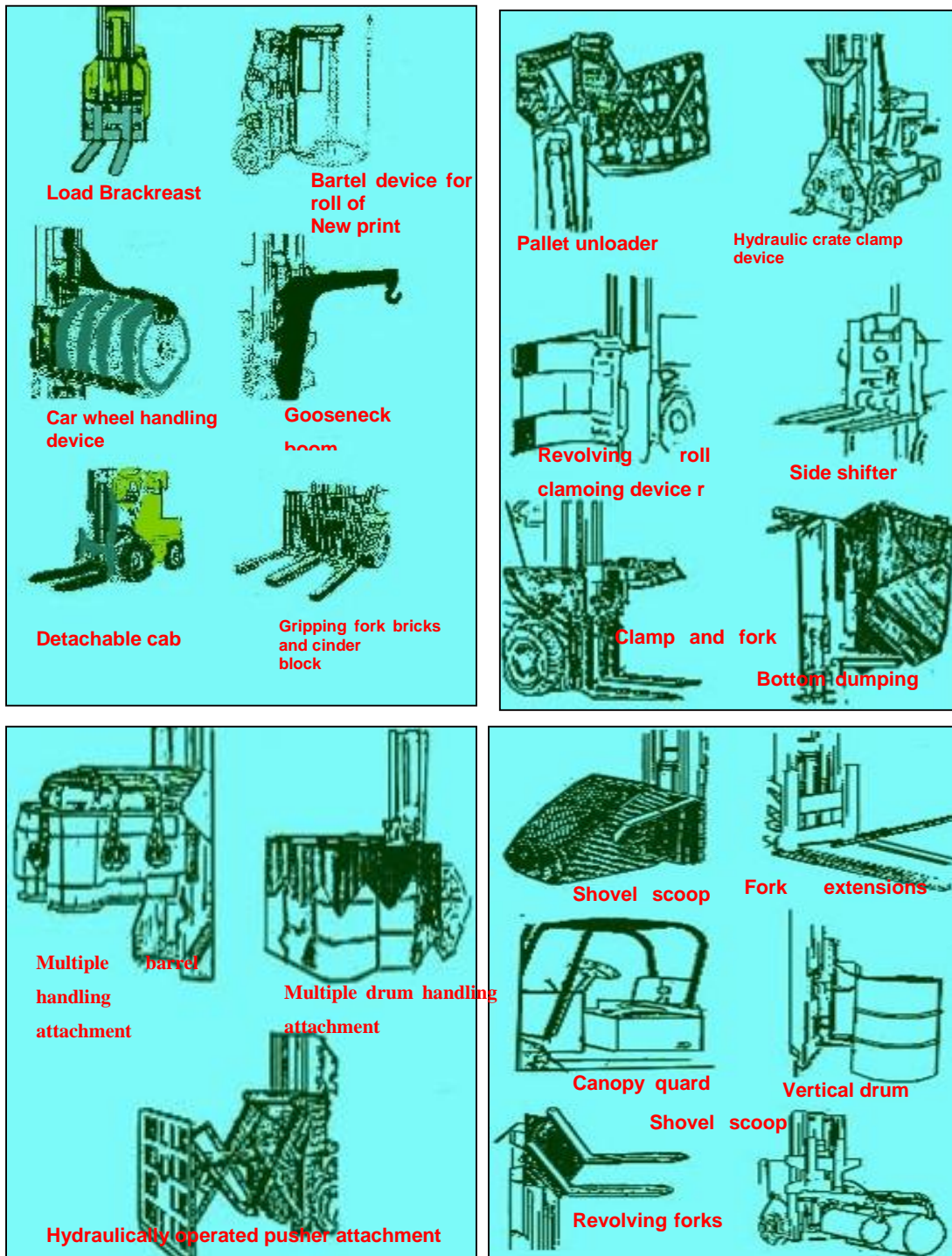
Gambar 21. Peralatan penunjang muat bongkar
