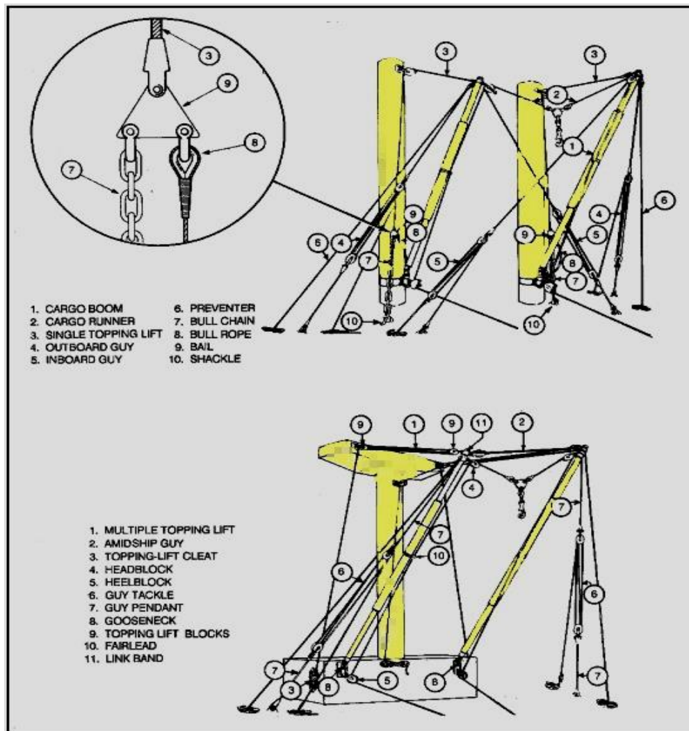
Gambar 4. Batang Pemuat Ganda Dengan Sistem Lopor Kawin Beserta Nama Bagian-bagiannya
