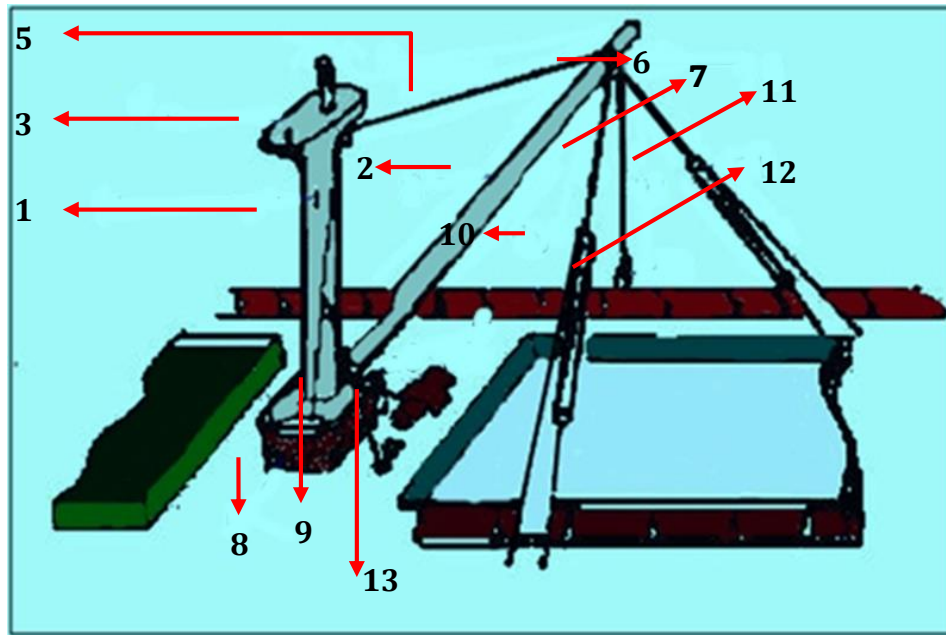
Gambar 1. Batang Pemuat Tunggal dan nama-nama bagiannya
