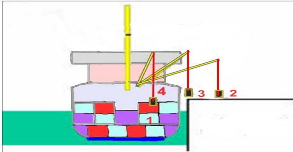
Gambar 26. Satu siklus bongkar muatan ( hookcycle time )
