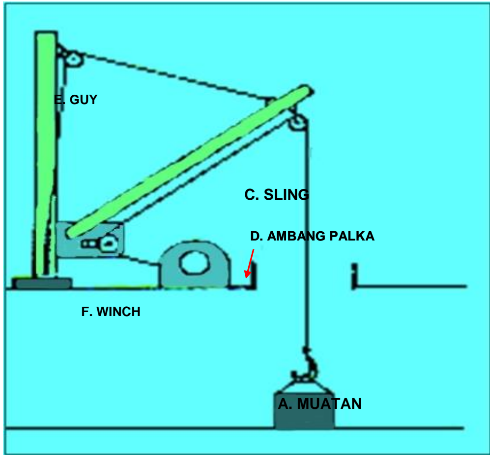
Gambar 3. Cara menggunakan batang pemuat
