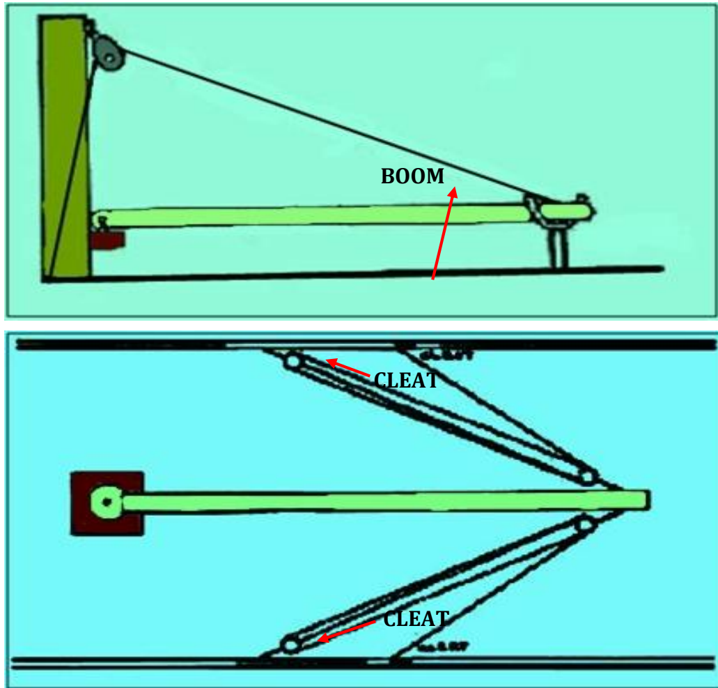
Gambar 2. Menyimpan batang pemuat saat kapal berlayar
