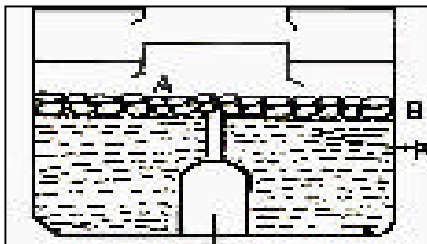
Gambar 31. Cara penyusunan muatan biji-bijian
