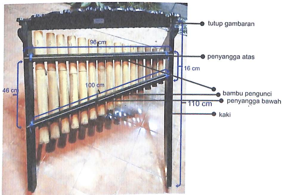
Ukuran rancak angklung paglak
