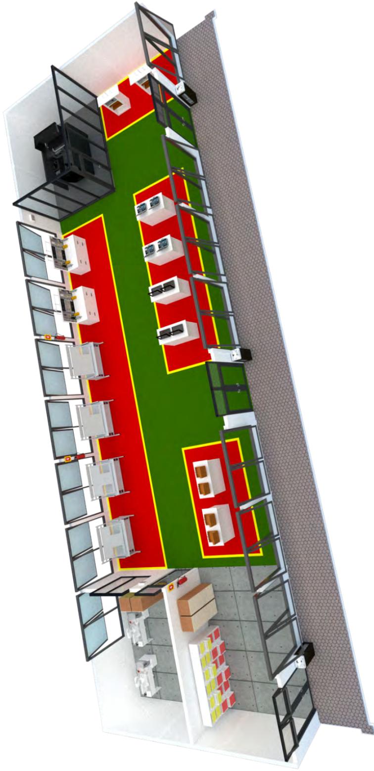
Gambar 22. Visualisasi 3D ruang praktik siswa kompetensi keahlian electrical avionics tampak 1
