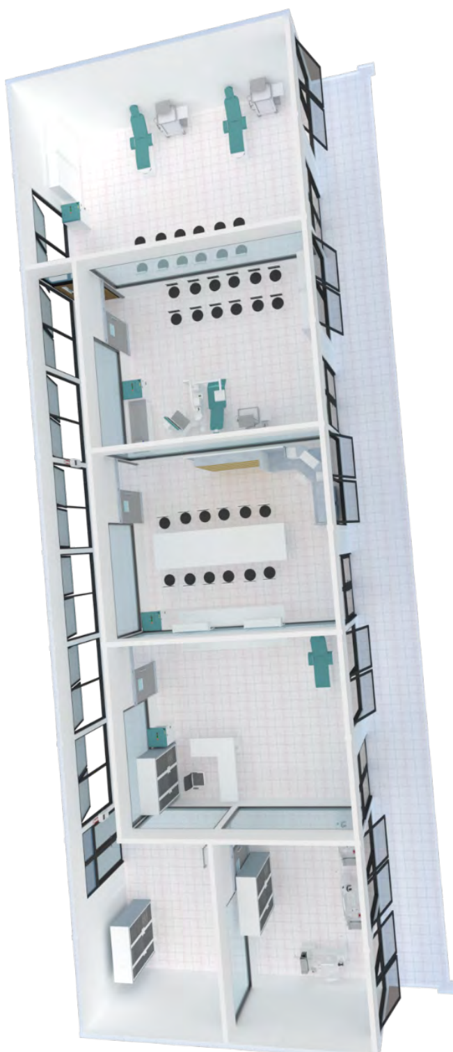
Gambar 22. Visualisasi 3D ruang praktik siswa kompetensi keahlian dental asisten tampak 1
