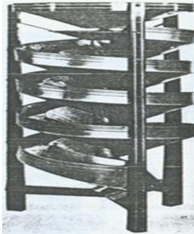
Gambar 18. Alat separator ulir
